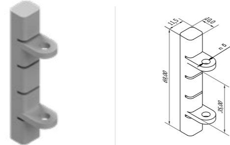
Deep Freezer Blowing Holder Part Derin Dondurucu Üfleme Yönlendirici Plastiği
