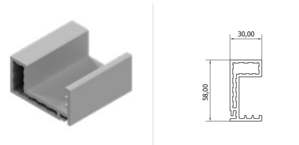
Deepfreeze Triple Glass Pillar Profile Derin Dondurucu Isıcam Dikme Profili
