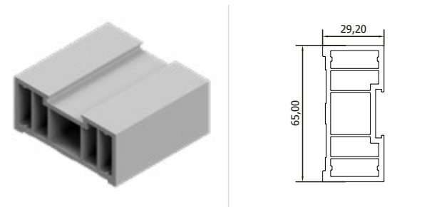
Frame Case Middle Pillar Profile Çerçeve Kasa Orta Kayıt Profili
