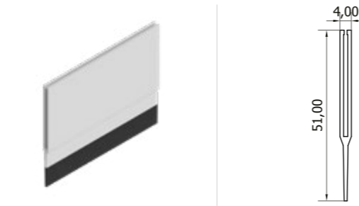
Flat Kick Plate Profile Düz Süpügelik Profili
