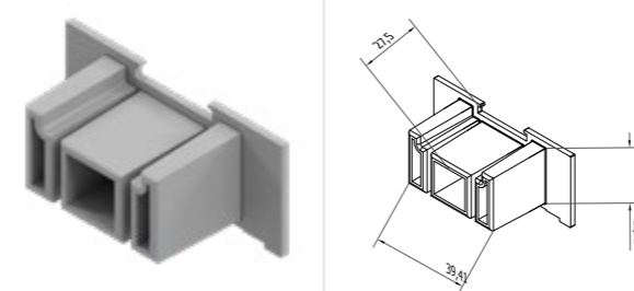
Frame Joining Wedge Çerçeve Birleştirme Takozu
