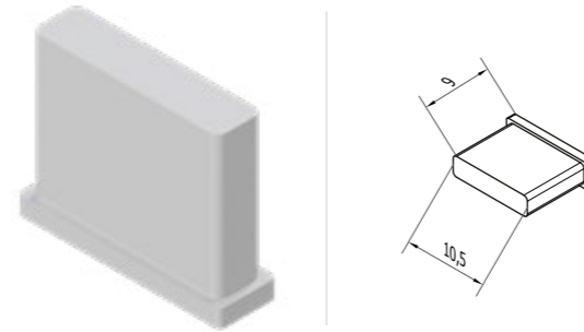
Magnetic Gasket Finishing Plastic Manyetik Conta Bitim Plastiği
