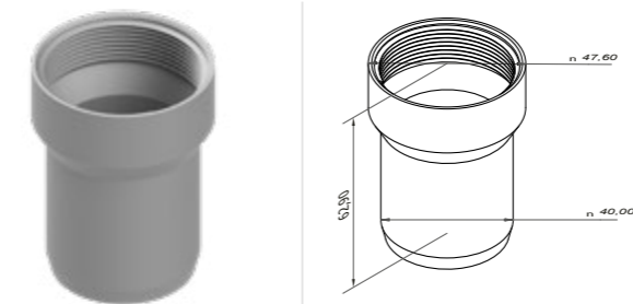
Water Drain Bottom Plastic Su Gideri Alt Enjeksiyon Plastiği
