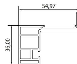
Gronied Frame Case Profile and Gasket Slot Çerçeve Pervazlı Kasa Profili ve Conta Yuvası
