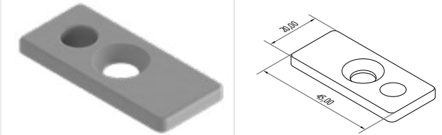
Frame Pin Socket Çerçeve Pim Soketi
