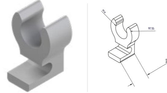
Pin Lock Plastic Pim Kilit Plastiği
