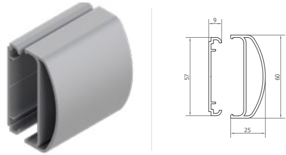
"D" Shape Bumper Profile + Mounting Bar "D" Tampon Profili + Montaj Çıtası
