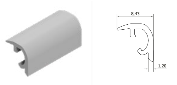
Sheet Metal Holder Clip Profile Sac Tutucu Kılıp Profili
