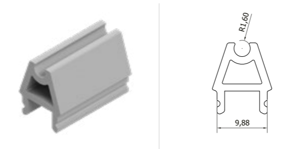
Heat Barrier Isı Bariyeri
