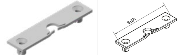
Frame Electrical Outlet Plastic Çerçeve Elektrik Çıkış Plastiği
