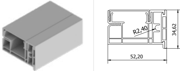
Industrial Kitchen Cabinet Body Profile Endüstriyel Mutfak Dolabı Gövde Profili
