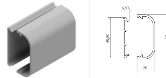
"U" Bumper Profile + Mounting Bar "U" Tampon Profili + Montaj Çıtası
