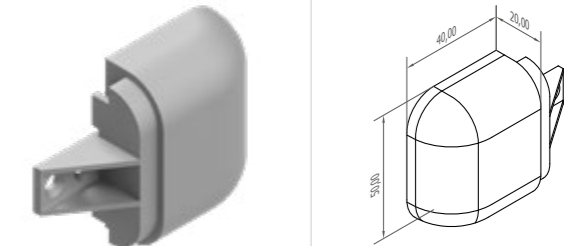
"U" Shaped Bumper Profile End Plastic "U" Tampon Profil Bitiş Plastiği
