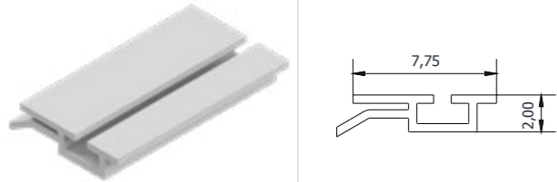
Gasket Holder Profile Conta Tutucu Profil
