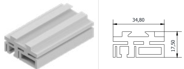
Gasket Holder Profile 2 Conta Tutucu Profil 2
