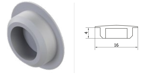
R12 mm Hole Plug R12 mm Delik Tapası
