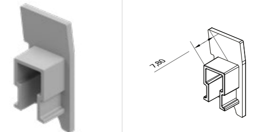
Semi Vertical Door Bottom Profile Cover Plastic Yarı Dikey Kapı Alt Profil Kapama Plastiği
