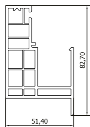
Frame Bottom Case Profile with Hinge Slot Çerçeve Menteşe Yuvalı Alt Kasa Profili
