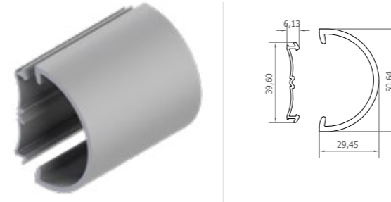
"C" Shaped Bumper Profile + Mounting Bar "C" Tampon Profili + Montaj Çıtası
