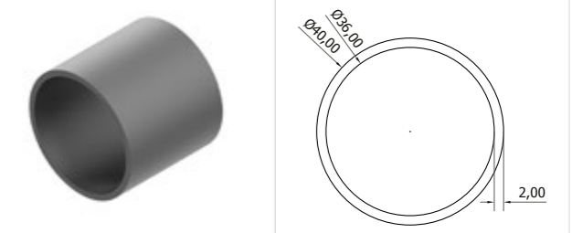
40mm Water Drain Pipe 40mm Su Gideri Borusu
