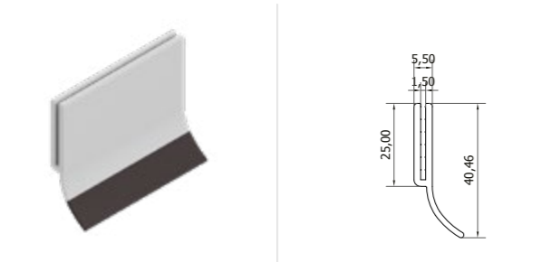
Radiused Kick Plate Profile Radüslü Süpügelik Profili
