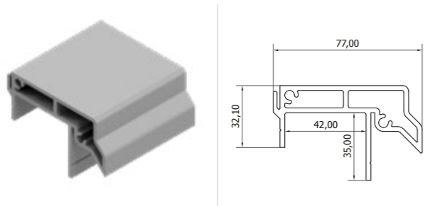
Body Frontal Profile Gövde Alın Profili
