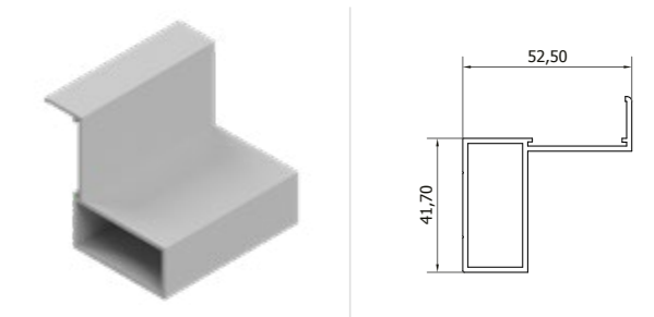
Groined Frame Case Profile Çerçeve Pervazlı Kasa Profili
