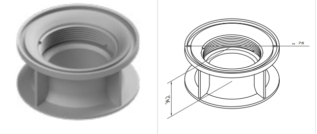
Water Drain Middle Plastic Su Gideri Ara Enjeksiyon Plastiği
