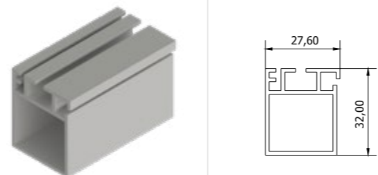
Industrial Kitchen Cabinet Door Profile Endüstriyel Mutfak Dolabı Kapı Profili
