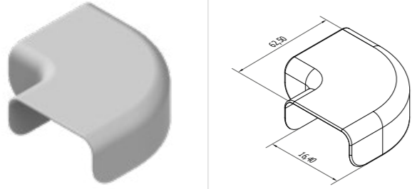
Hand Rail Corner Part El Rayı Köşe Dönüş Plastiği
